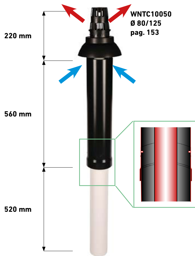
Installazione su tetti piani con tegola N5-TN13
